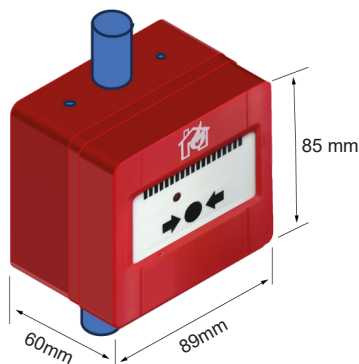
Caja instalación para superficie
