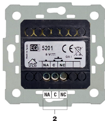
2 Contactos de salida. Output contacts.
